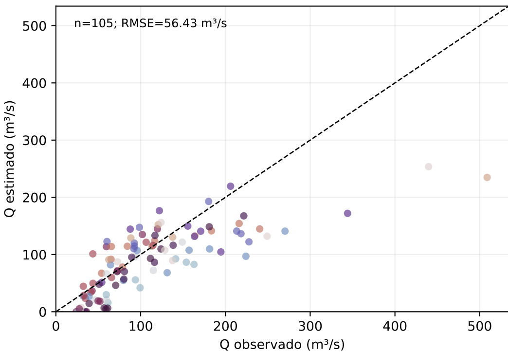
IMERG · validación de desarrollo
