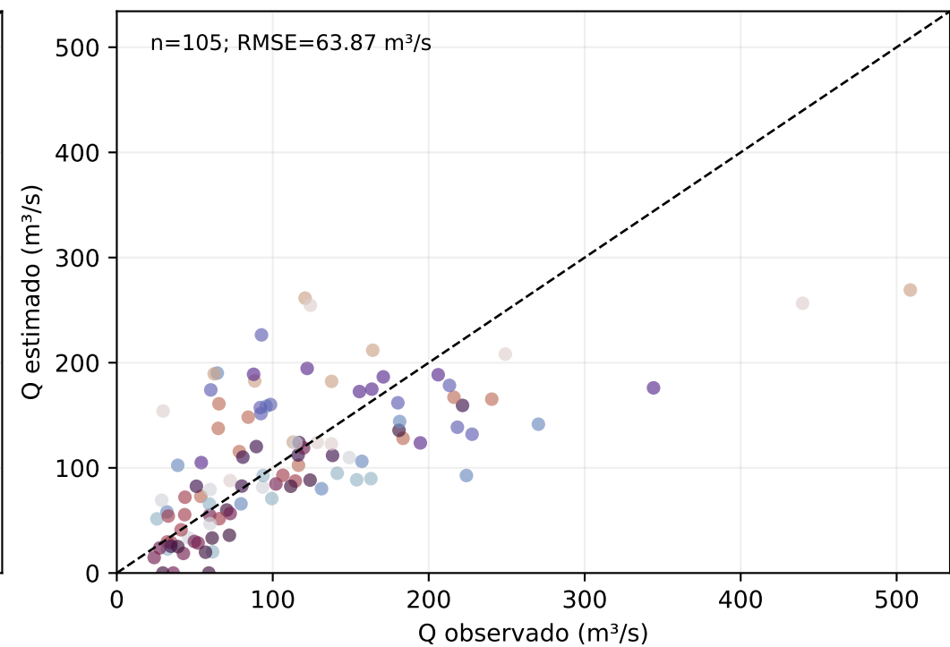
CHIRPS · validación de desarrollo
